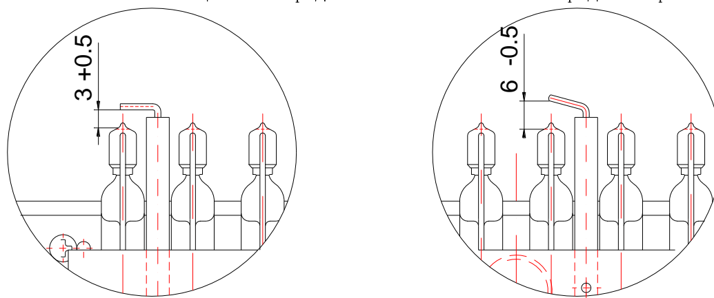
Рис. 6.1.2.1. Расположение электрода в горелке
