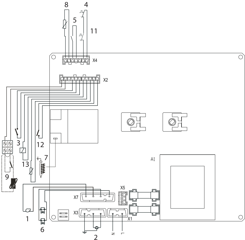
Рис. 11. Принципиальная электрическая схема
