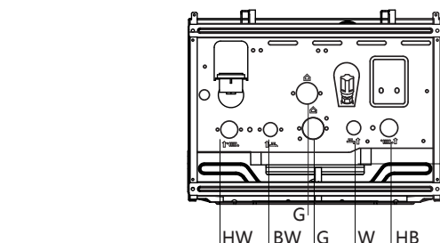
Пластиновый теплообменник
