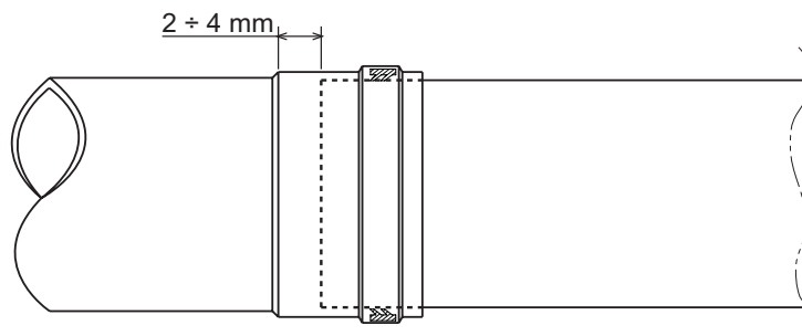
рис. 20 - Тепловое расширение
