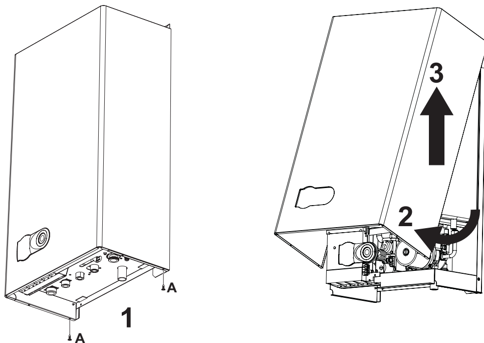
рис. 16 - Снятие кожуха
