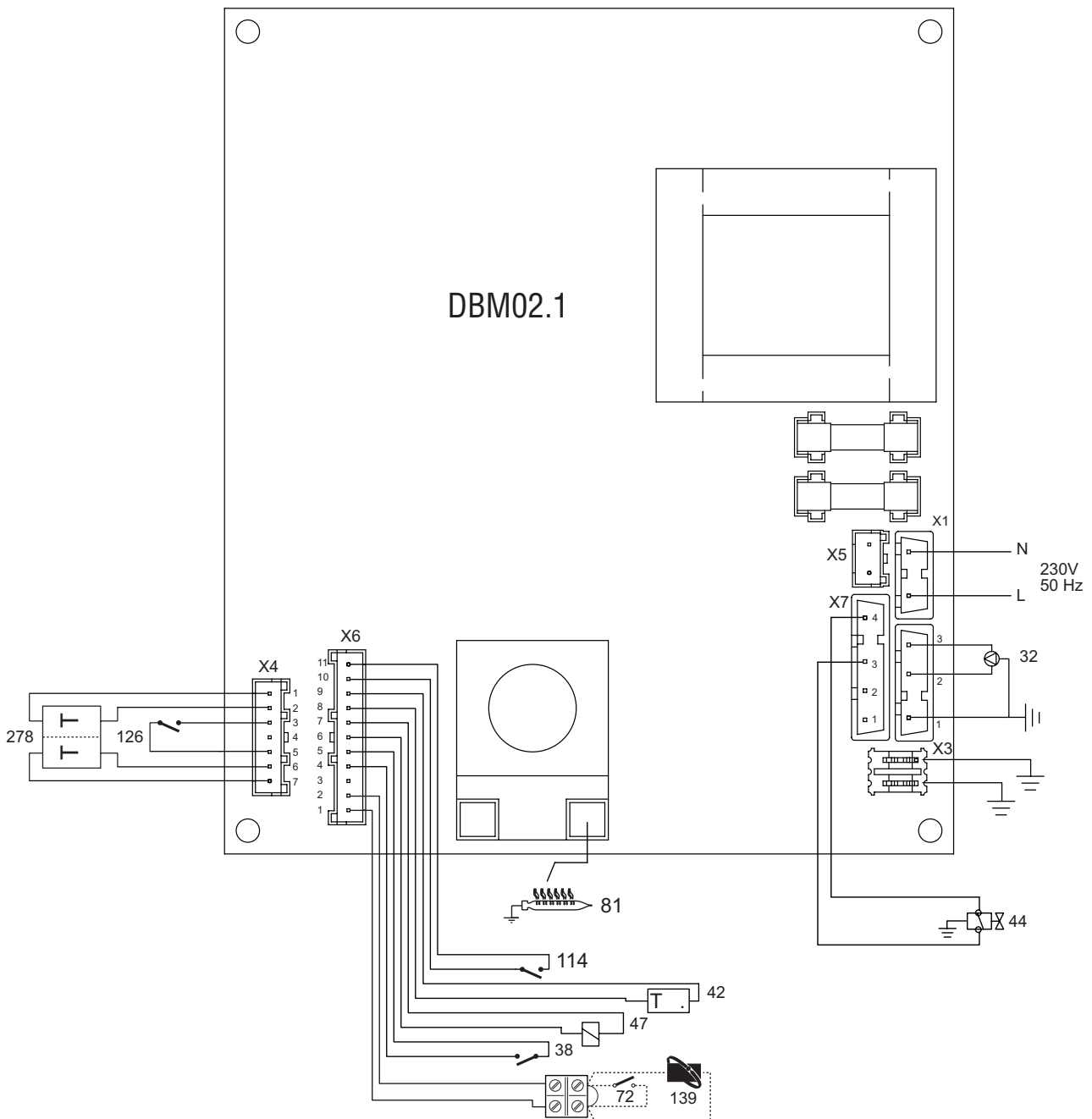
рис. 20 - Электрическая схема
