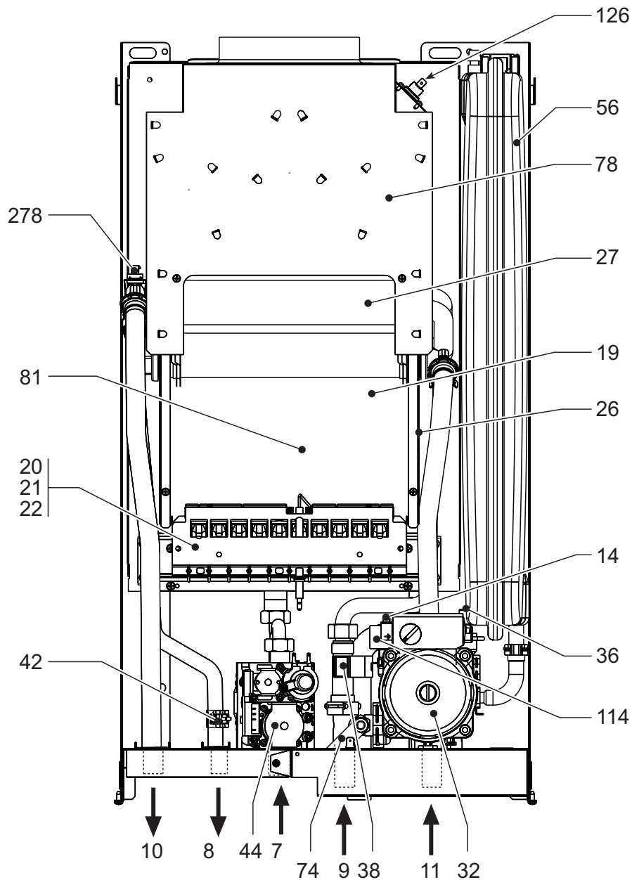
рис. 18 - Общий вид
