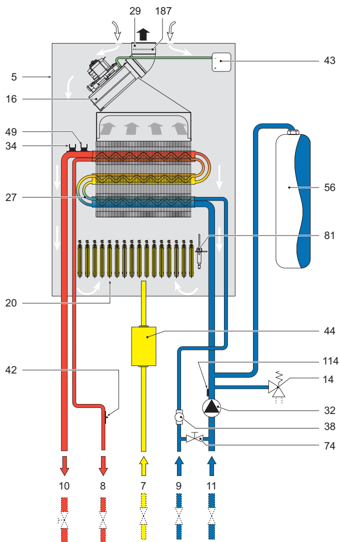
рис. 21 - Схема системы отопления и контура ГВС
