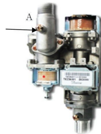
Рисунок 14. Газовый узел
