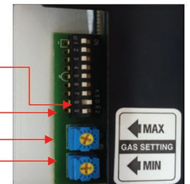
Рисунок 15. DIP-переключатели
