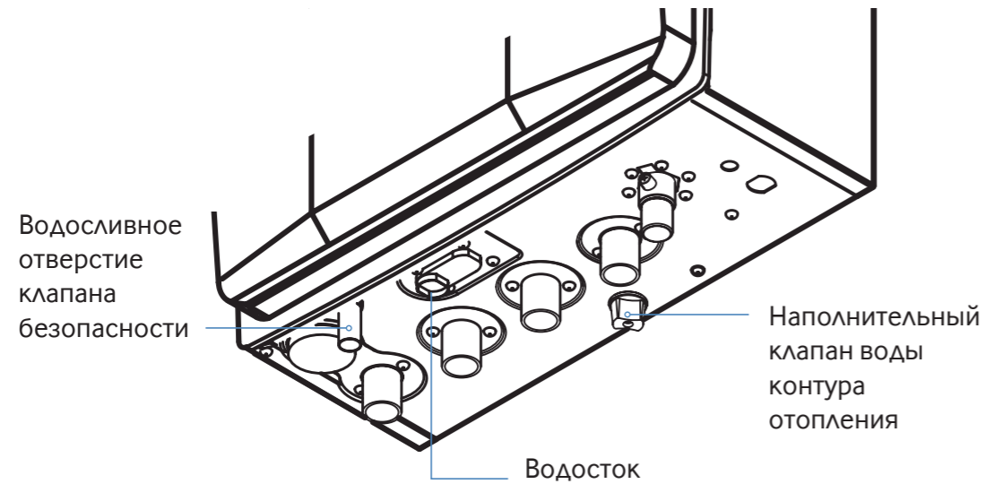
Рисунок 8. Схема нижней панели
