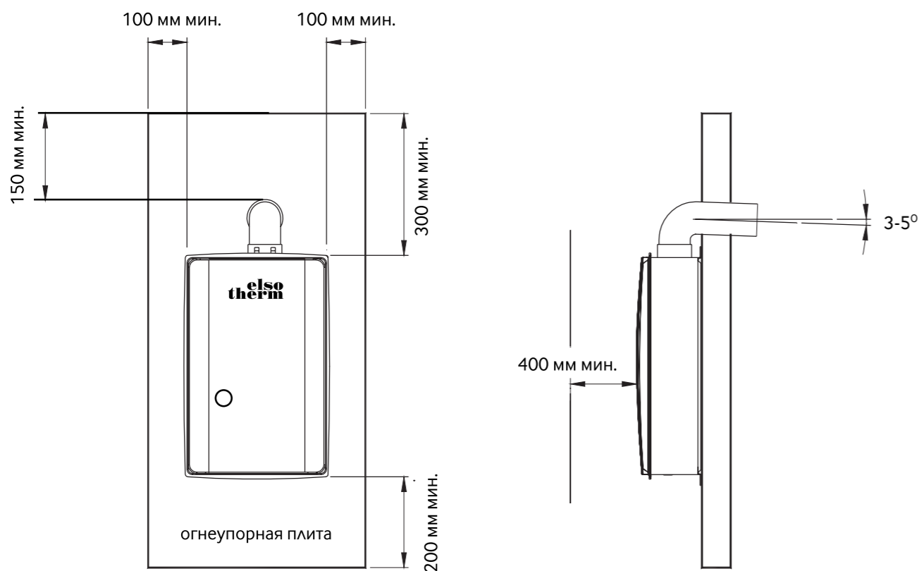
Рисунок 11. Установка котла
