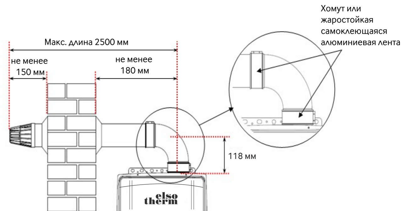
Рисунок 12. Установка дымохода
