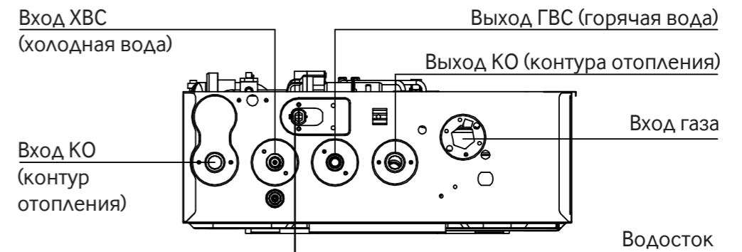
Рисунок 1. Устройство и назначение основных частей
