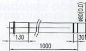
DGB-S1000 (Труба прямая 1000 мм.)
