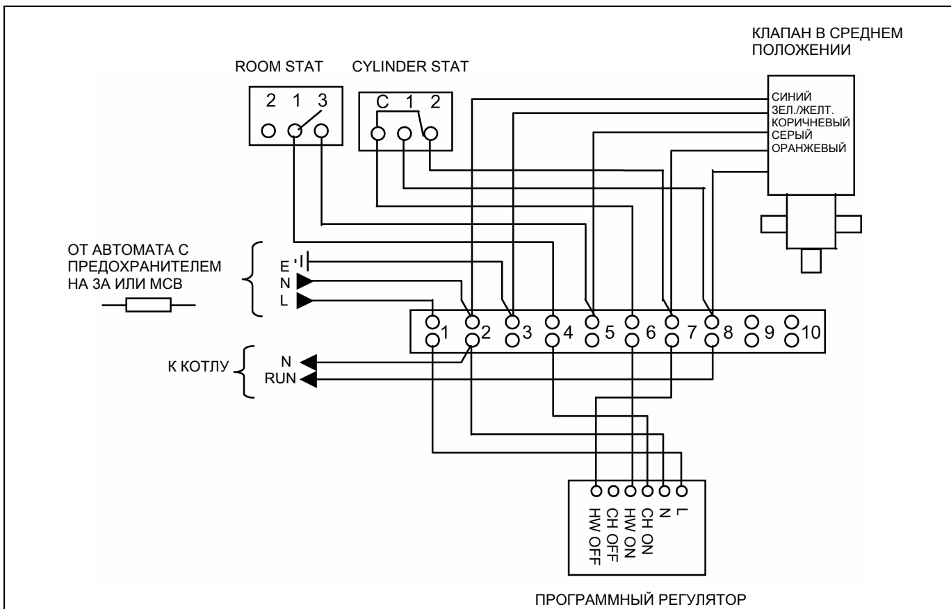
РИС. 9 ТИПИЧНАЯ ЭЛЕКТРИЧЕСКАЯ СХЕМА Y PLAN
