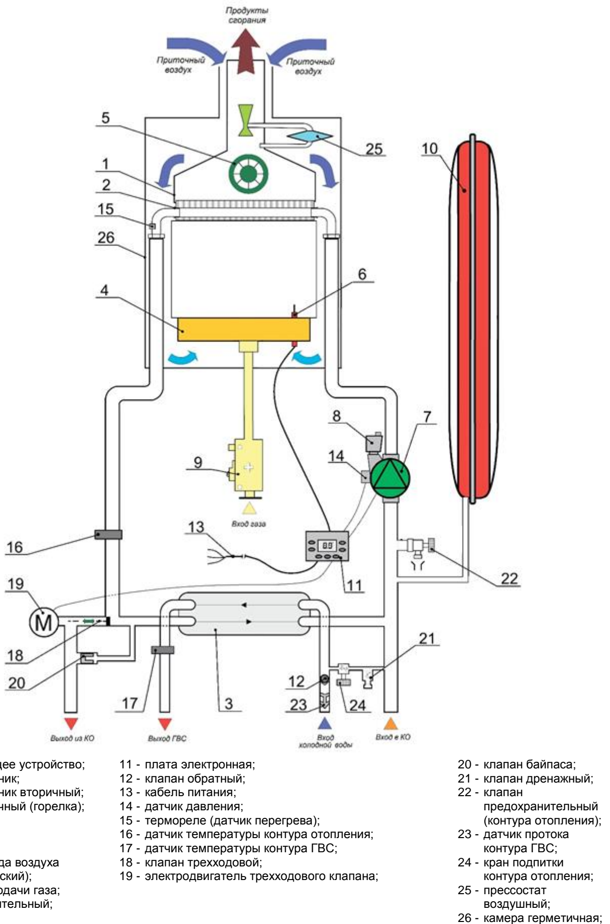
Рис. 7 Функциональная схема котла
