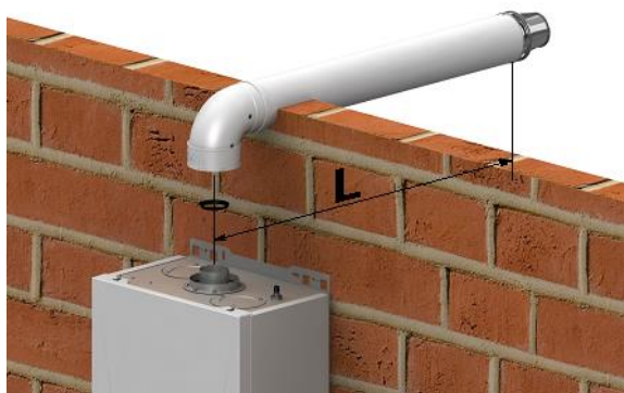
Рис. 3 Схема присоединения коаксиального дымохода Ø 100 / Ø 60 (мм) к котлу и установка диафрагмы
