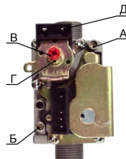
Рис. 6 Регулятор подачи газа
